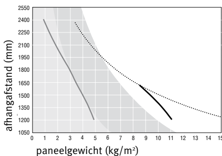
C 600 x 1800 standaard
