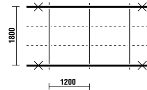
D 600 x 1200 kruisverband 1800 h.o.h.
