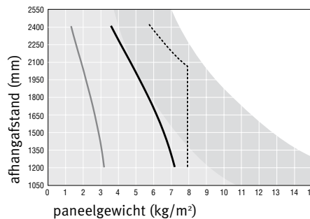
D 600 x 1200 kruisverband 1800 h.o.h.
